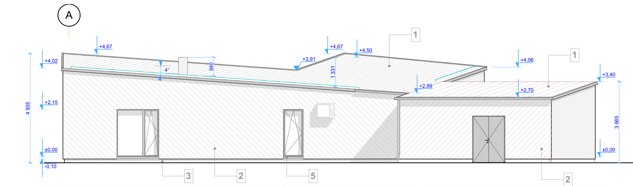
E-22 (= telg 5) VAADE KIRDEST 1:100
