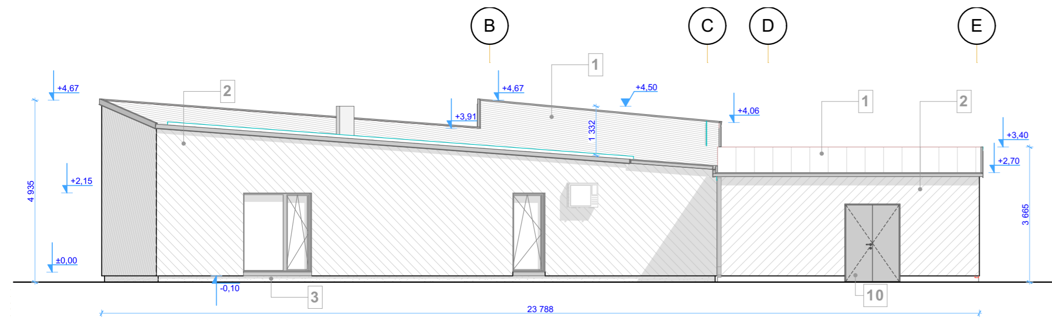
E-12(=telg 1) VAADE KIRDEST 1:100
