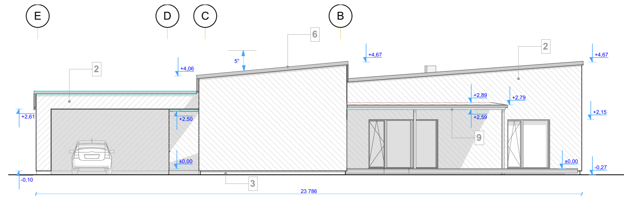
E-14 (=telg 1) VAADE EDELAST 1:100
