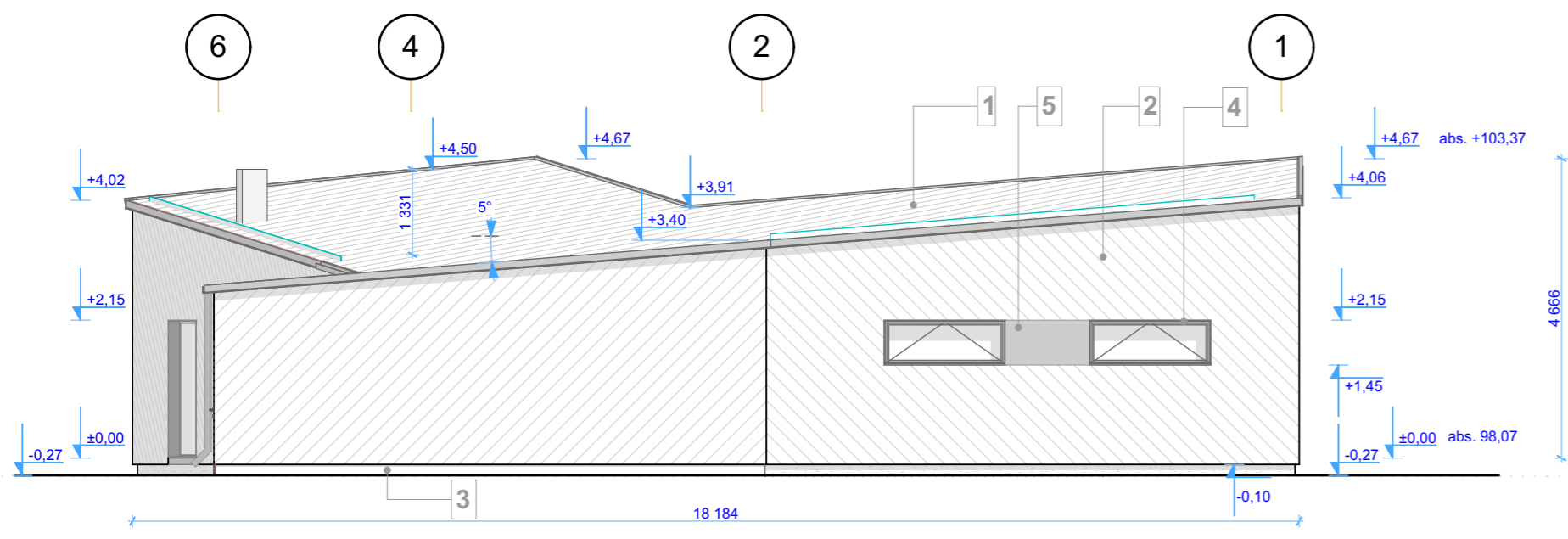
E-11 (=telg E) VAADE LOODEST 1:100
