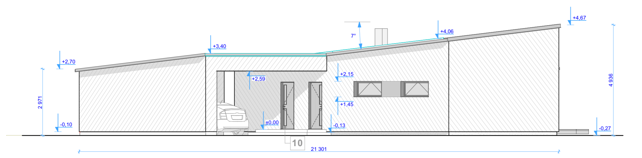
E-34 (=PKK) VAADE LÄÄNEST 1:100
