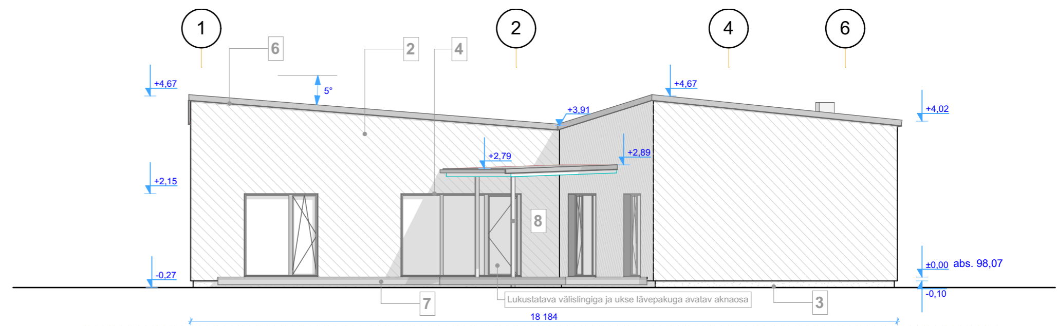
E-13 (=telg C) VAADE KAGUST 1:100
