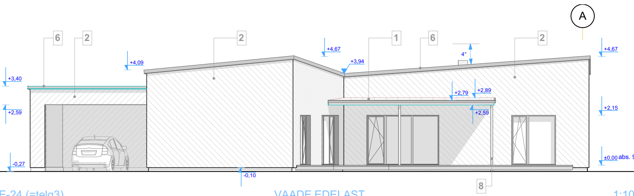
E-24 (=telg3) VAADE EDELAST 1:100
